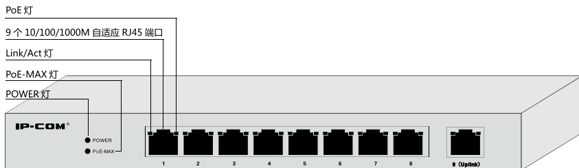
图 1-1 前面板
