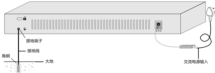
图 2-5 机房附近允许埋设接地体时接地安装简图
